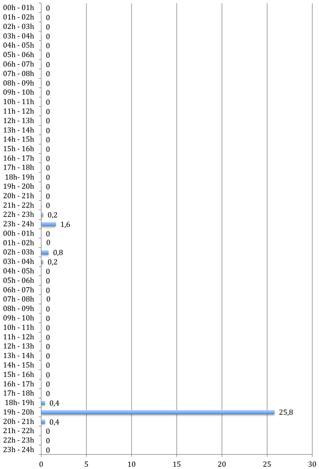
Cantidades de lluvia registradas por horas en SEDAVÍ los días 15 y 16/09/21 (en l/m 2 )
